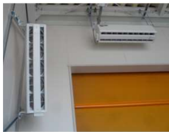
2重シートシャッターとエア搬送ファン
